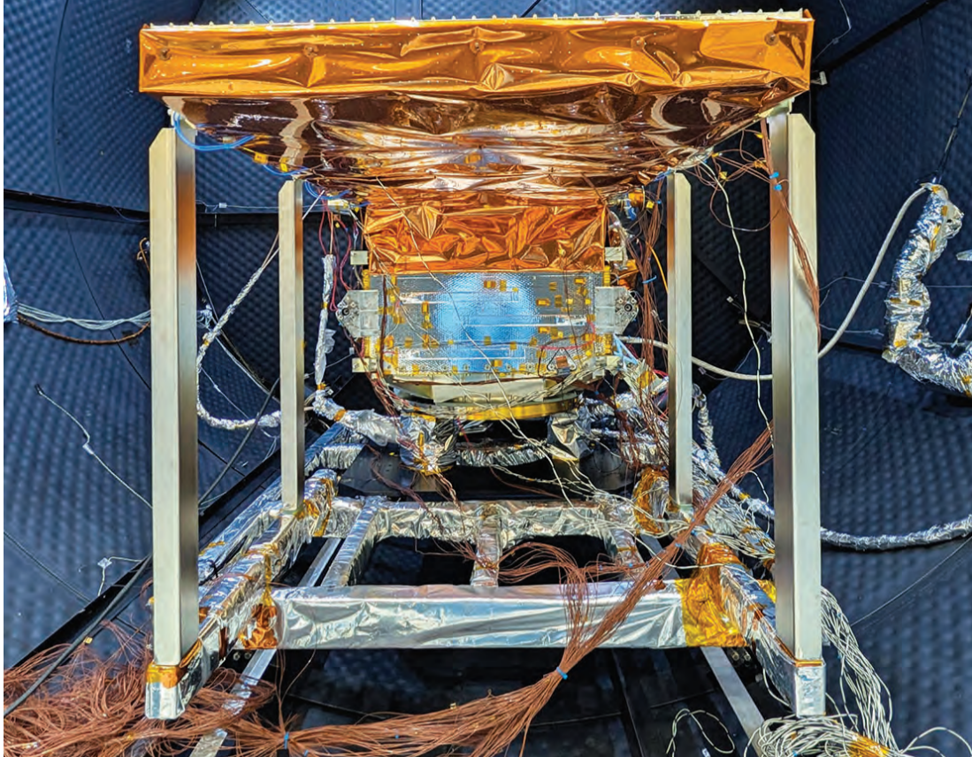
القمر الاصطناعي «الاتحاد سات» الأول من نوعه المزود بتقنية التصوير الراداري | من المصدر
